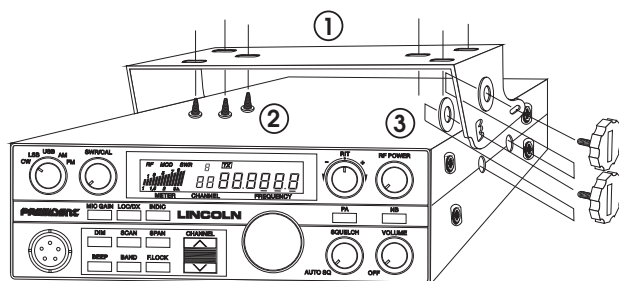
SCHEMA GÉNÉRAL DE MONTAGE
